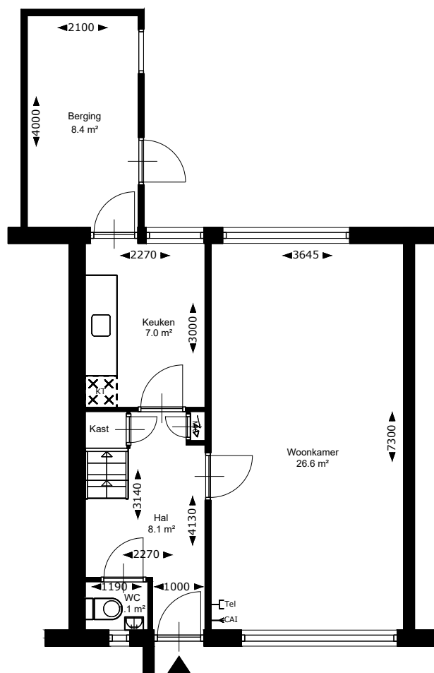
Begane grond
