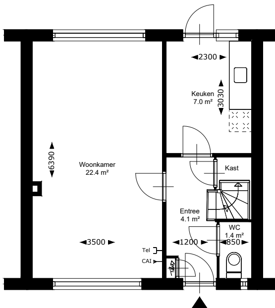
Begane grond
