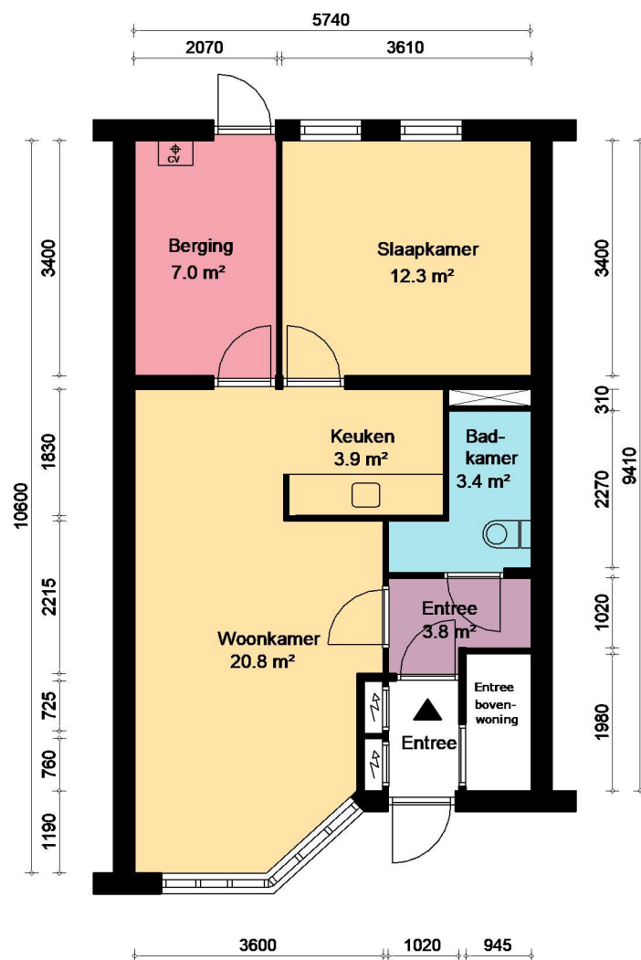
Begane grond
