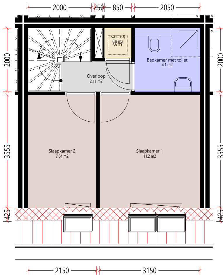
Verdieping_1e
