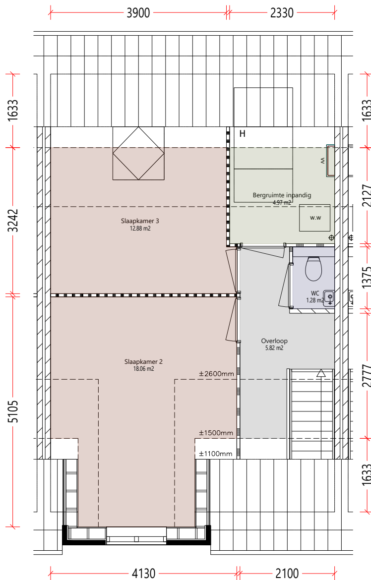
Verdieping_1e
