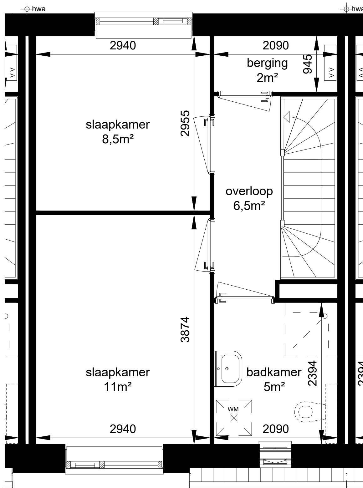
Eerste verdieping
