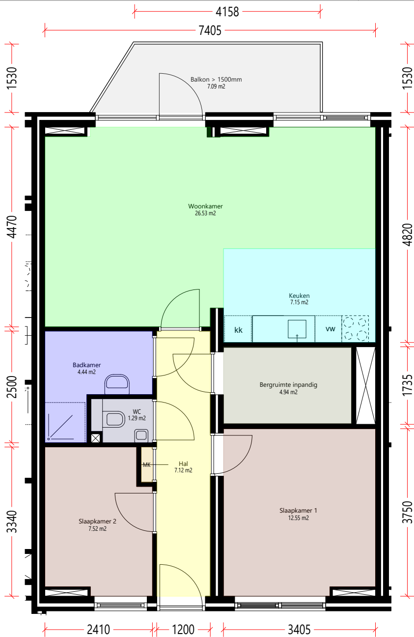
Verdieping_1e
