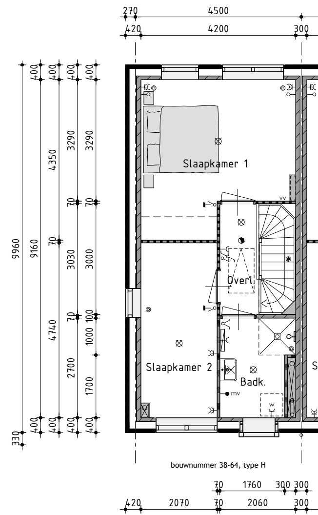
1ste Verdieping
