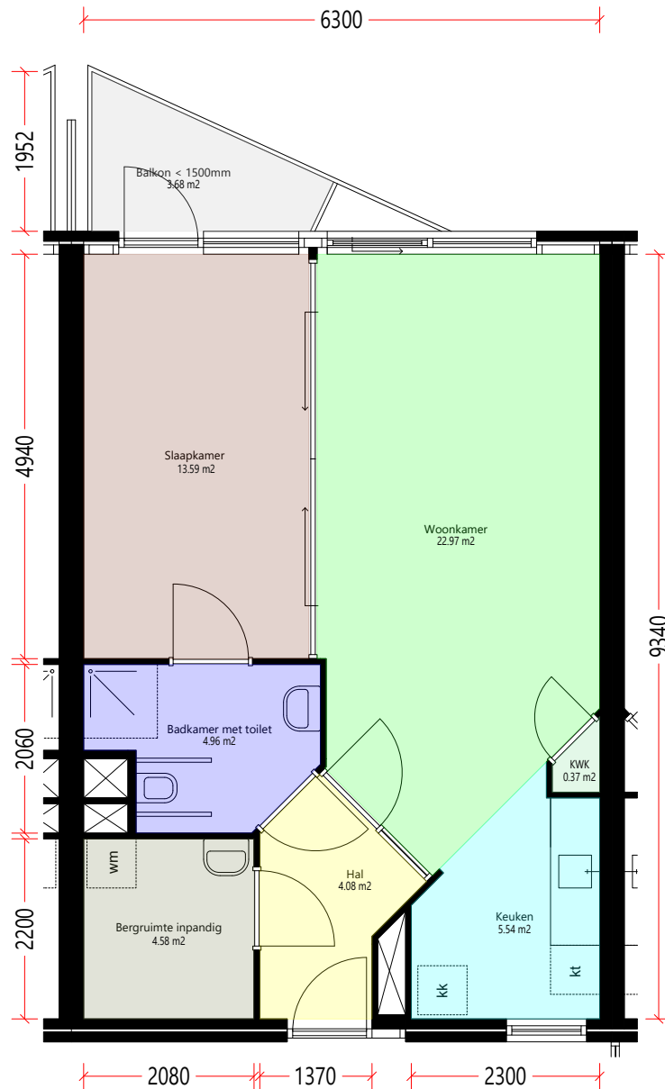
Verdieping_1e
